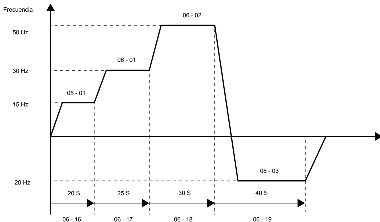
Figura 11.2.1 Operación automática de un solo ciclo (Paro)
